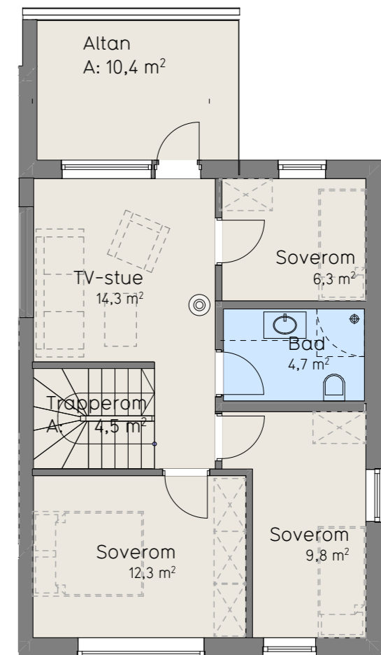
1:100 2. Etasje
