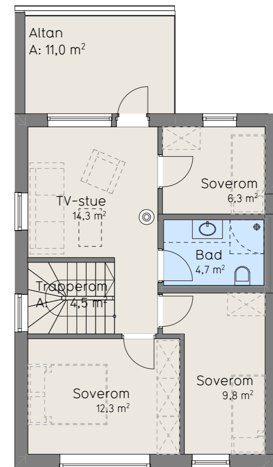
1:100 2. Etasje
