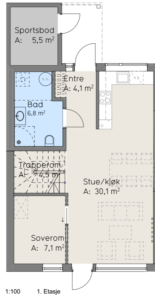
1:100 1. Etasje
