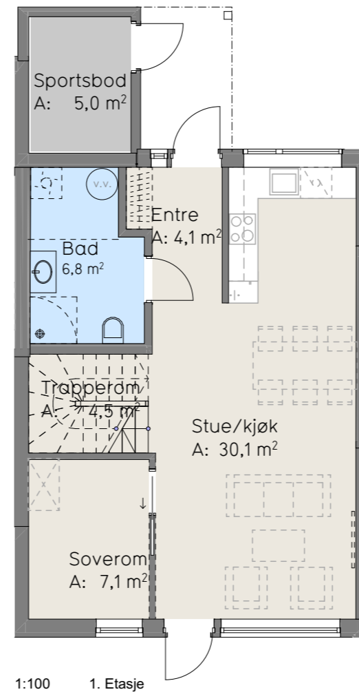
1:100 1. Etasje
