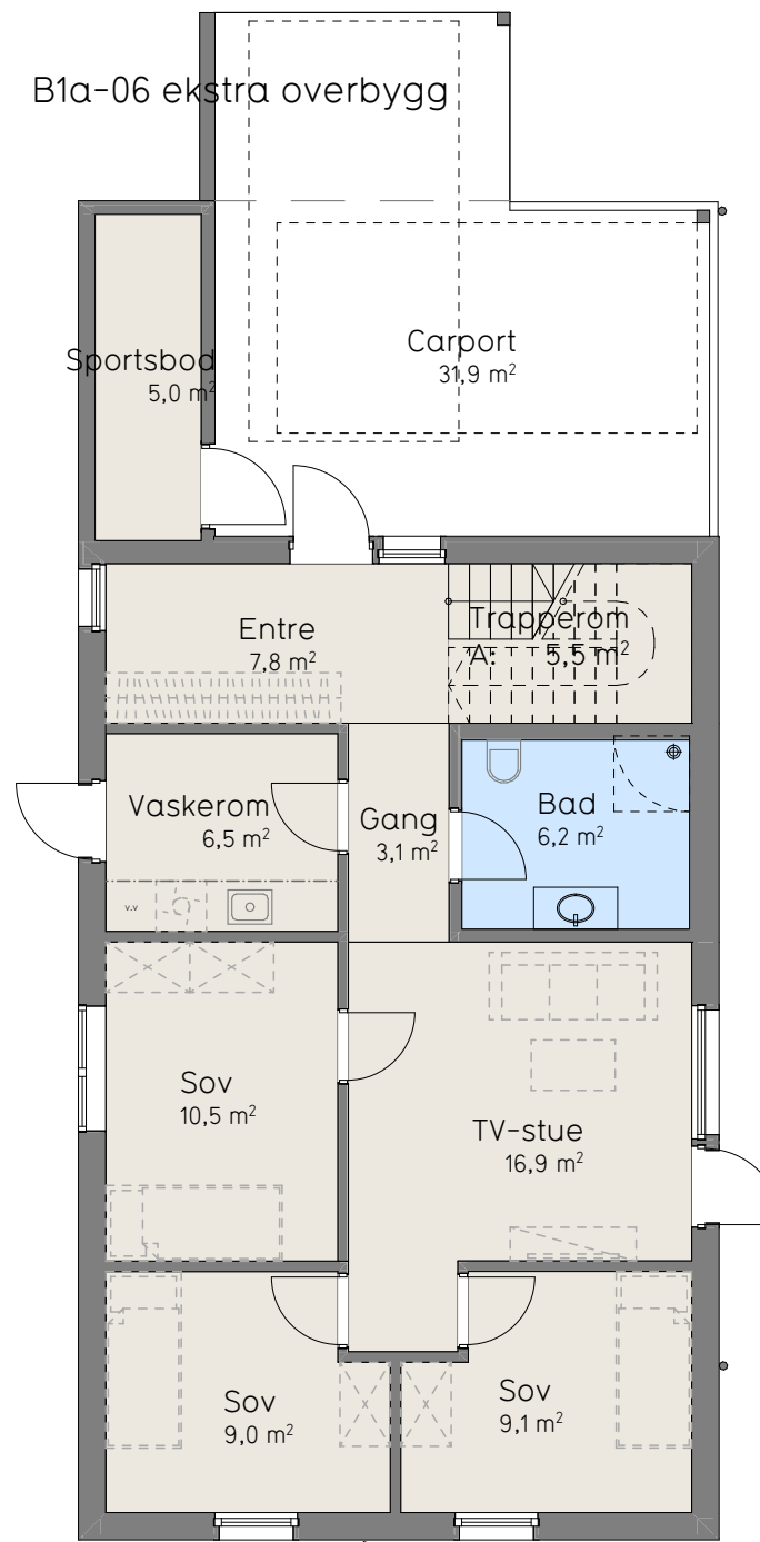
1. Etasje enebolig 1:100
