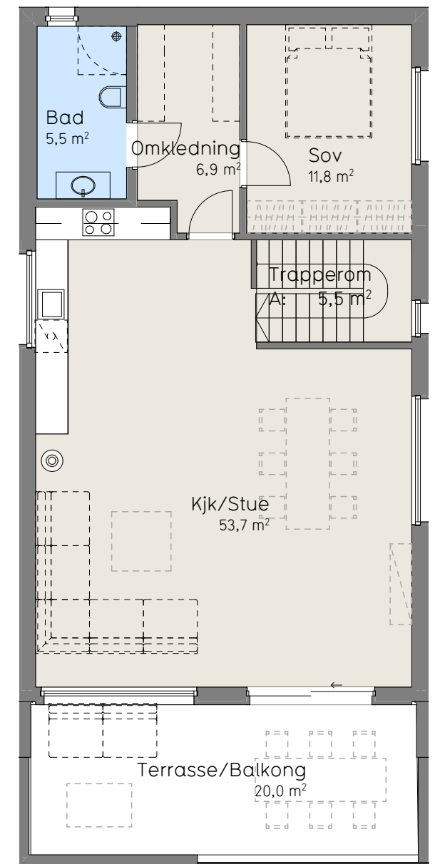
2. etasje enebolig 1:100
